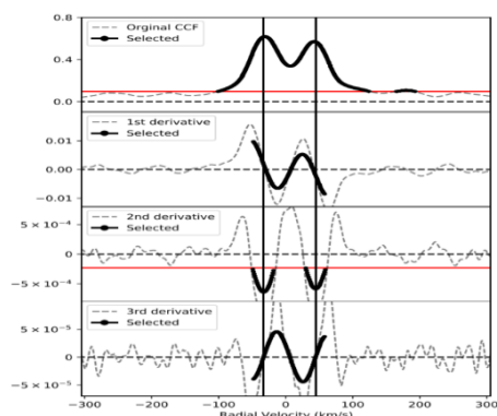
图 1 双星系统中两颗子星的视向速度变化
